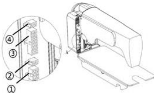
Рис.1-1 Схема гнезда контрольного блока
