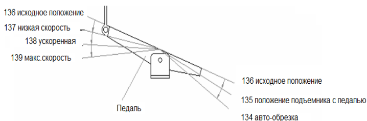
Рис. 4-1. Перемещение педали для каждого параметра положения
