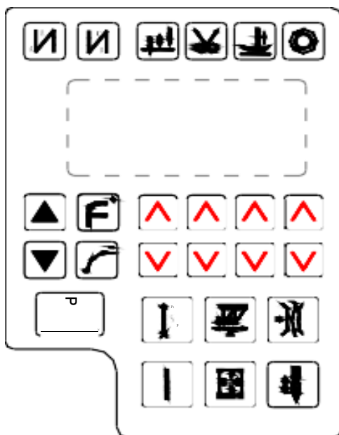
Рис.2-1. Панель управления
